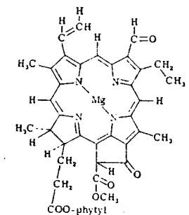
Chlorophyll b
